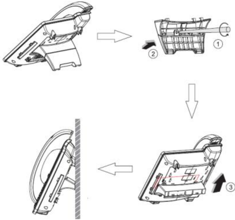
图 2 - 壁挂式话机安装
