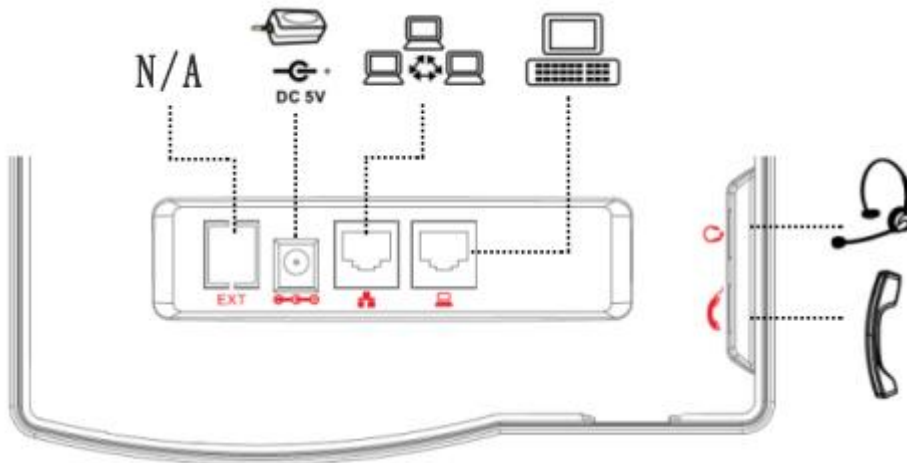
图 3 - 设备连接
