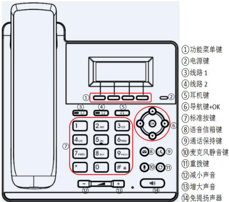
图 4 - 按键说明
